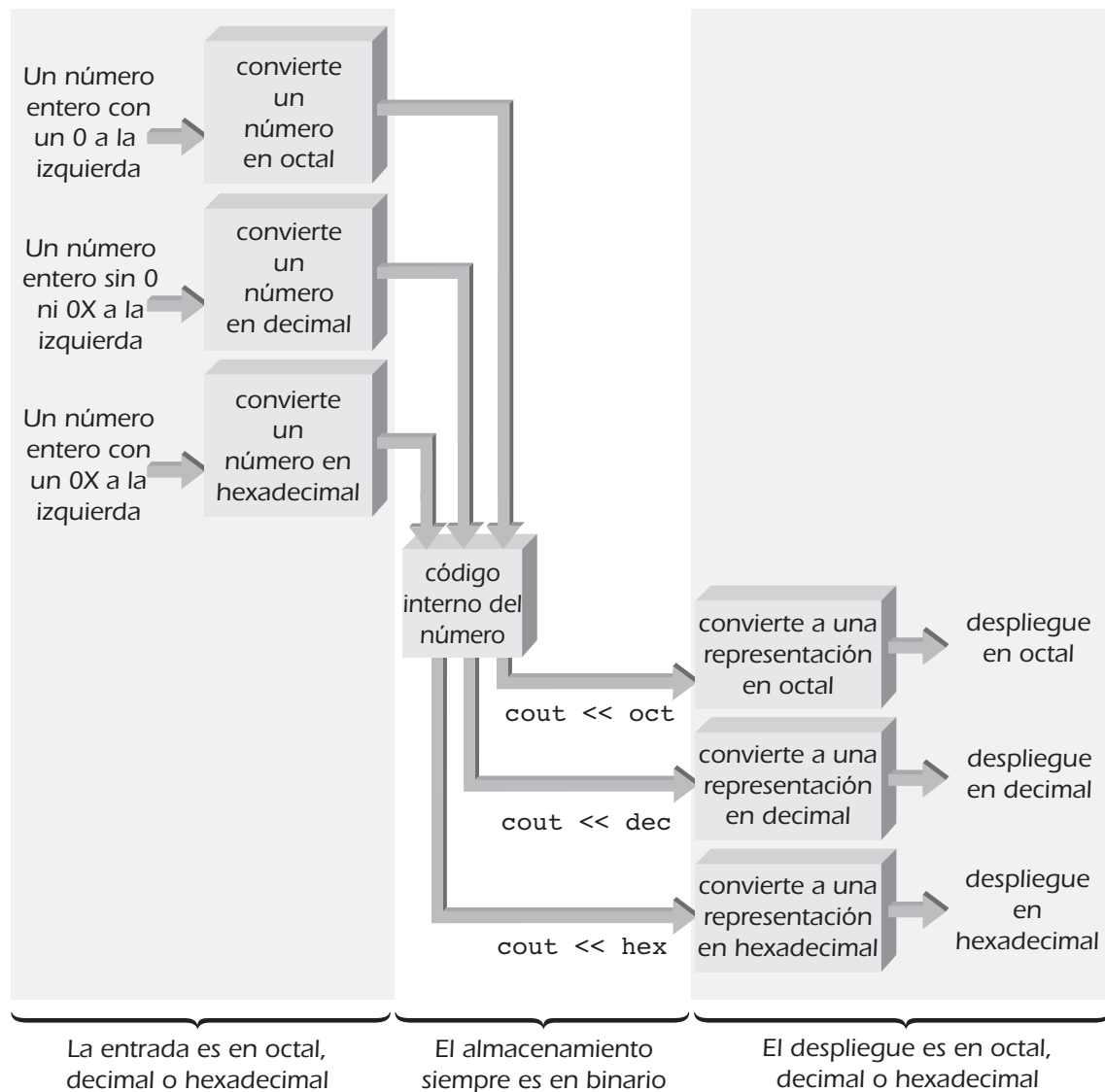
Figura 3.8 Entrada, almacenamiento y despliegue de números enteros.
