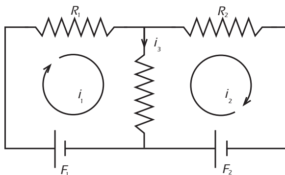
Figura 3.7 Un circuito eléctrico.
